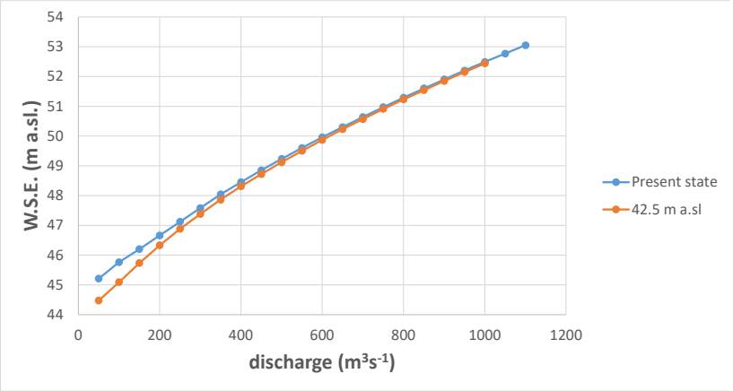
Figur 1. Vannstands-vannføringskurve ved utløp av Vangsvatnet for nåværende tilstand og med senkning av utløpsterskel til kote 42.5 moh.
