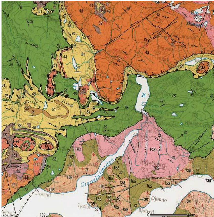
Figur 5. Geologisk berggrunnskart for Granvin herad (Kjelde: www.ngu.no)
